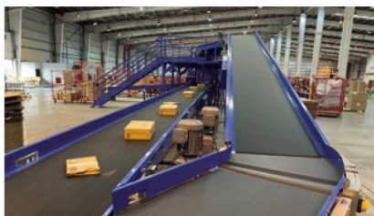
Los paquetes se clasifican en función de su destino a través de las múltiples salidas en ambos niveles.
