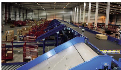
Sistema de clasificación construido a dos niveles por JHernando para la plataforma de Coslada de Sending.
